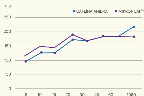
Figura. Concentrações da Cafeína Anidra e Mikroncaf™ no plasma.
